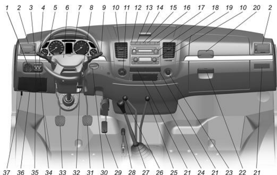
Obr . 5.1. Palubní deska a ovládací prvky
