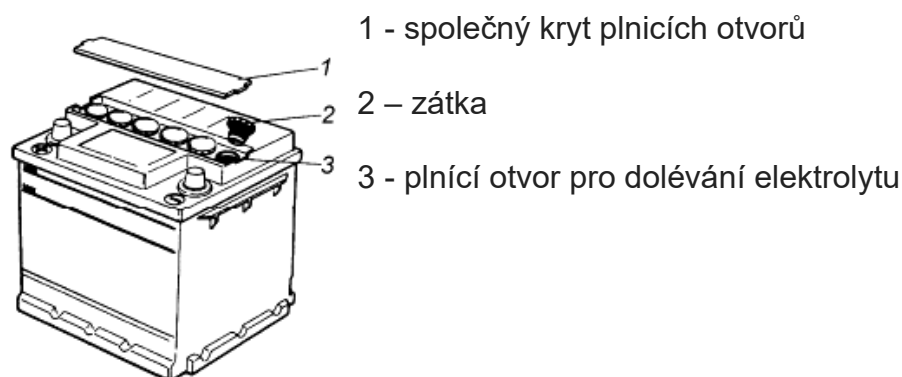
Obr. 9.5. Baterie:
