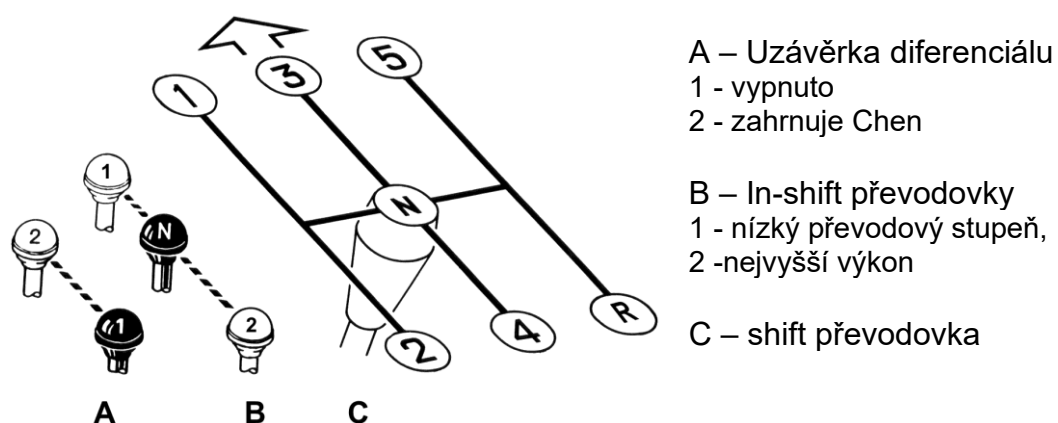
Obr. 5.18. Schéma řazení:
