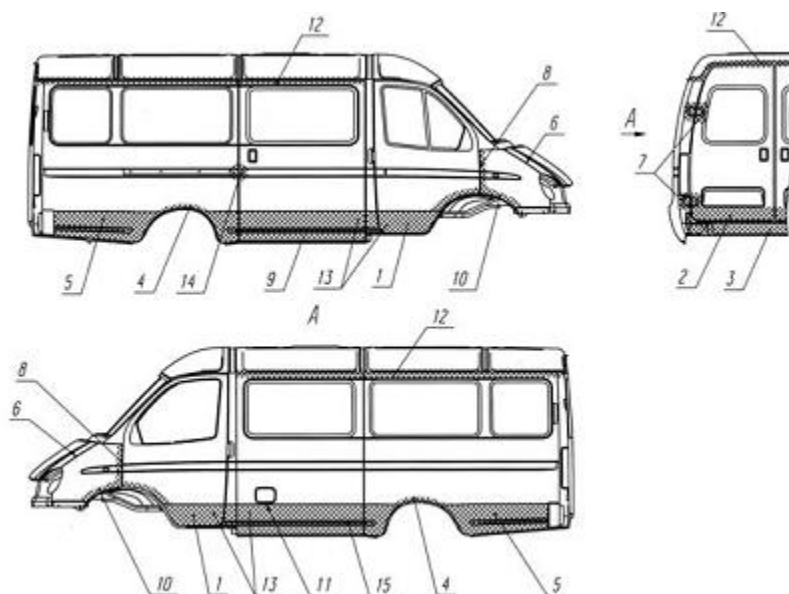
Obr. 9.9 Schéma antikorozičního ošetření dutin a kabiny vyžadující zvýšenou péči
